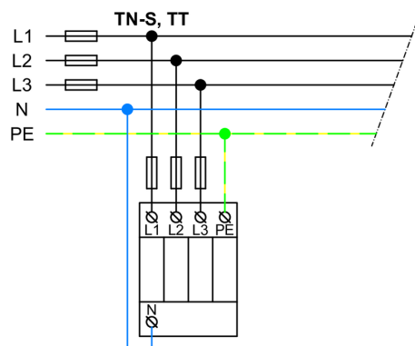
Aplikační schéma zapojení (instalace)
