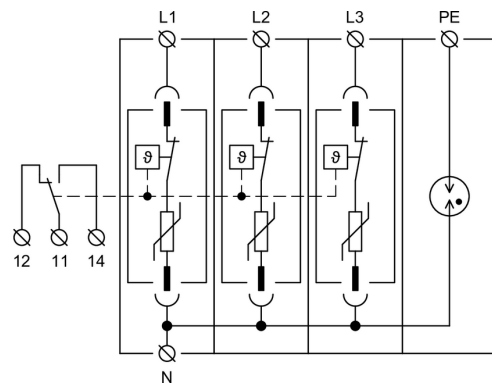
Vnútorná schéma zapojenia
