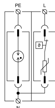
Vnútná schéma zapojenia
