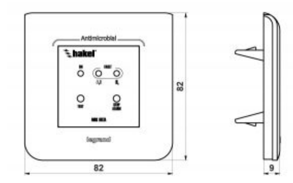
Rozměrový výkres
