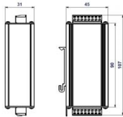
Rozměrový výkres
